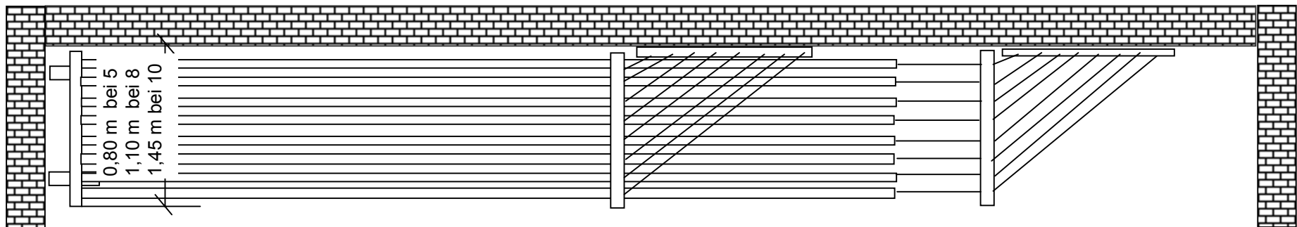
Einbauskitze für Schrägtrocknungs – anlage STK Doppelanlage mit einer Aufhängekapazität von 5/ 8 / 10 C und 5 / 8 / 10 B Schläuchen !
