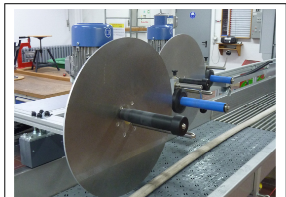
(Schlauchwicklersystem EW2)
